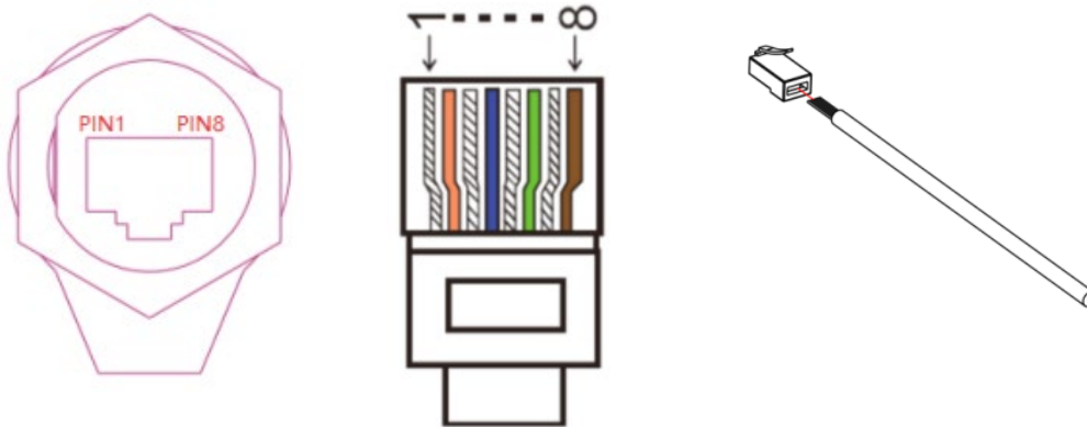
Figura 185 - Collegamento interfaccia DRMs (1)
