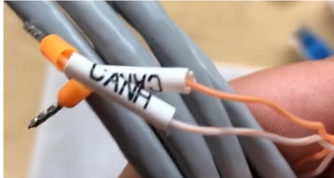
Figura 105 - Cavo comunicazione Inverter/HV BOX
