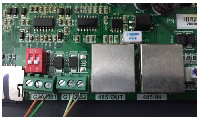
Figura 256 - Collegamento linea seriale tramite morsetteria RS485 e tramite plug RJ45
