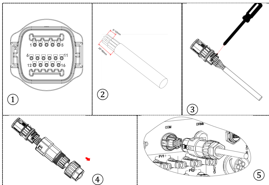
Figura 96 - Connessione porta COM "a incastro"
