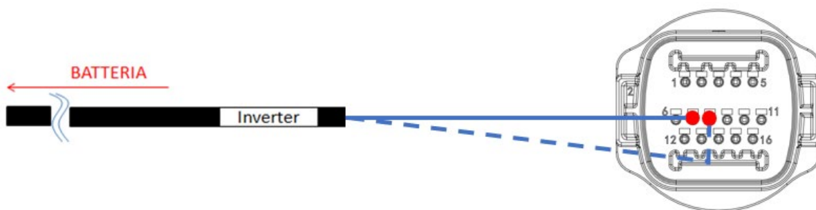
Figura 160 - Schema connessioni COM "a incastro"
