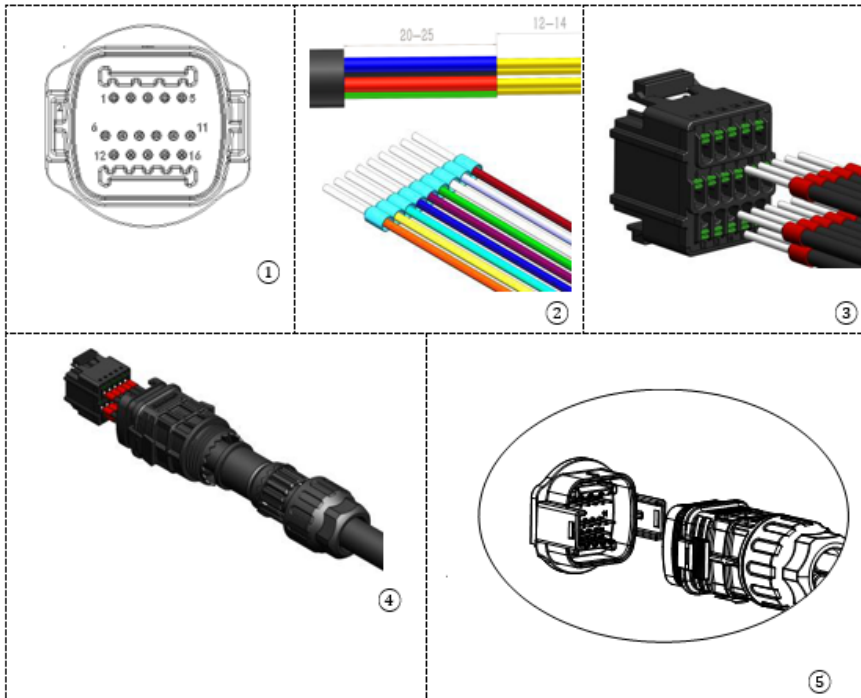
Figura 95 - Connessione porta COM "a vite"
