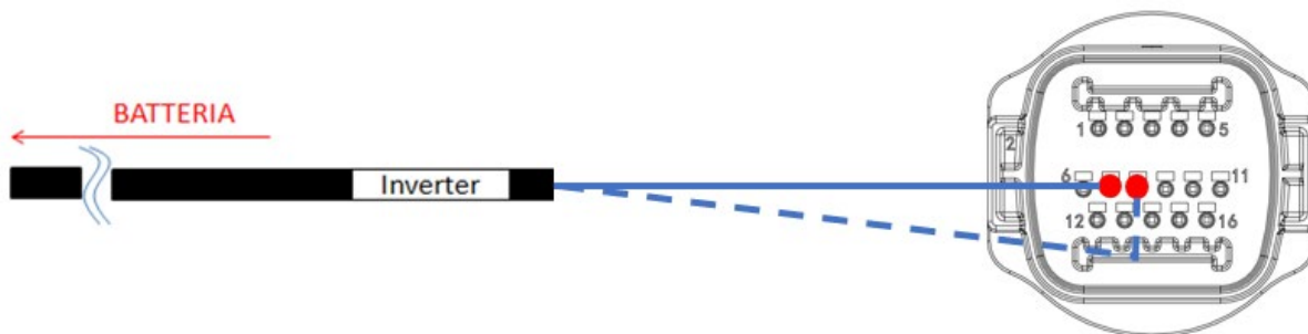
Figura 179 - Schema connessioni COM "a incastro"
