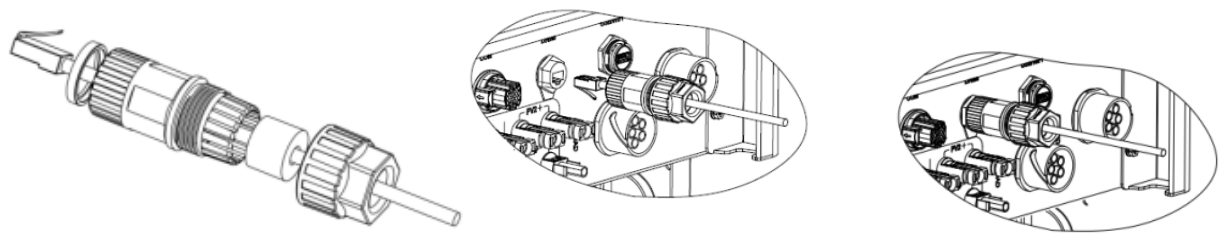
Figura 186 - Collegamento interfaccia DRMs (2)
