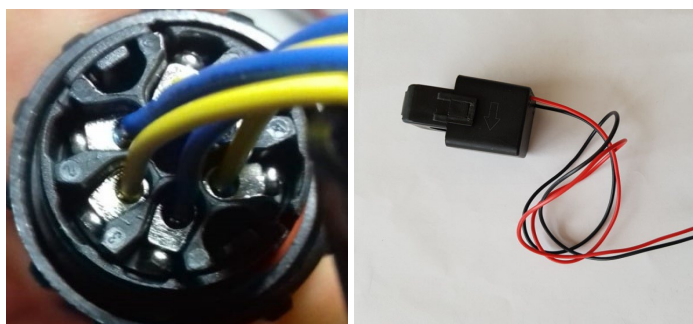
Figura 190 - Collegamenti numerati connettore CT
