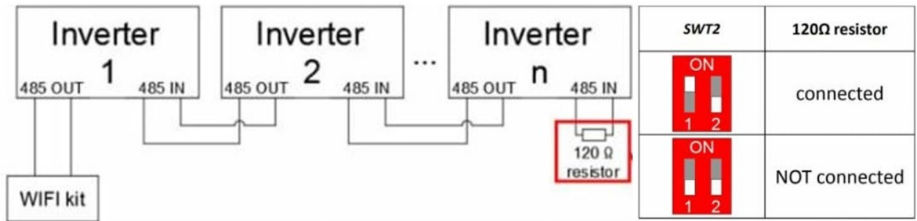
Figura 260 – Posizione dei dip switch per collegare la resistenza di isolamento
