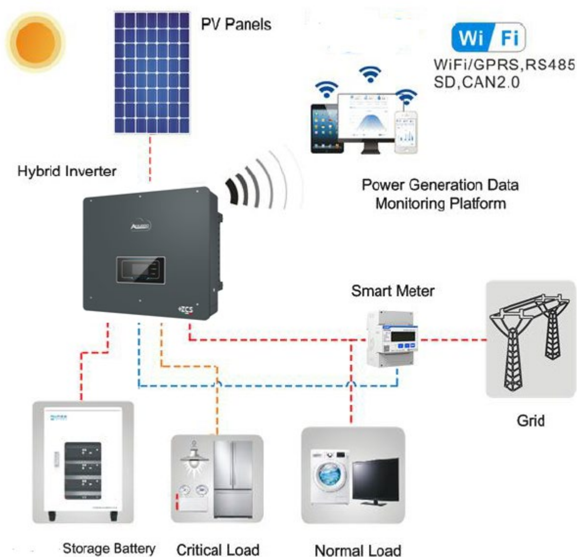
Figura 1 - Diagramma schematico di un impianto con inverter ibrido 3PH HYD5000-HYD20000-ZSS
