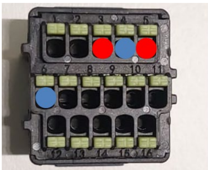
Figura 259 - Collegamento della linea seriale tramite connettore di comunicazione per 3PH HYD5000-HYD20000-ZSS
