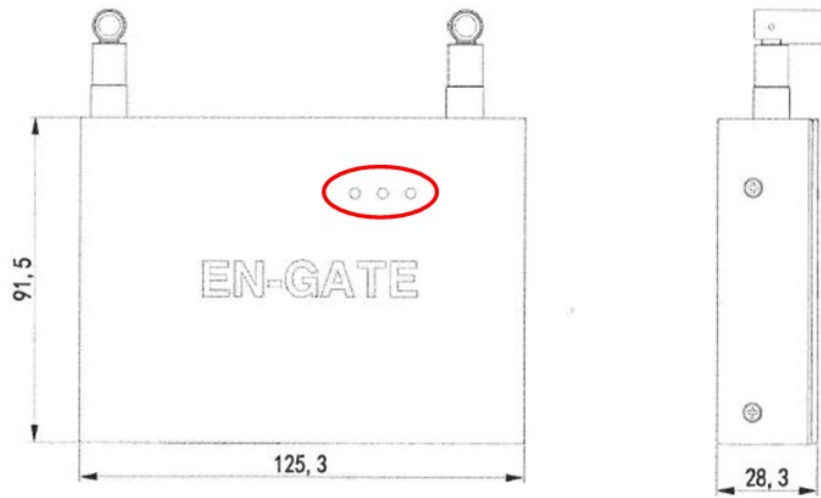
Figura 40 - Dimensioni dispositivo
