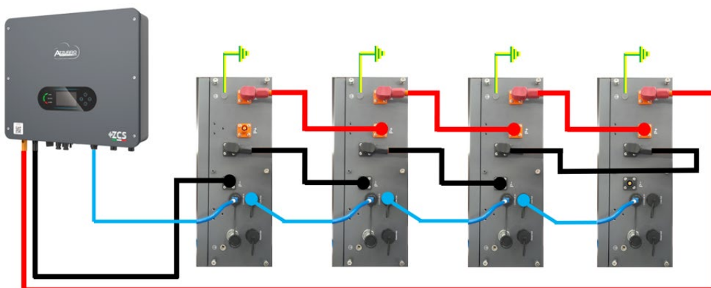
Connexion de 4 batteries
