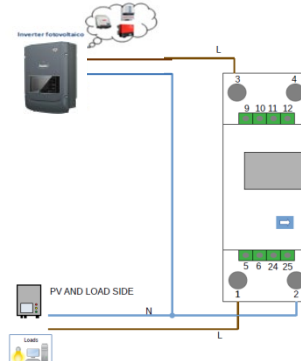
Meter sur Production Extérieure
