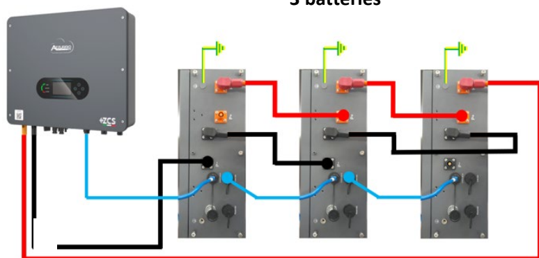
Connexion de 3 batteries
