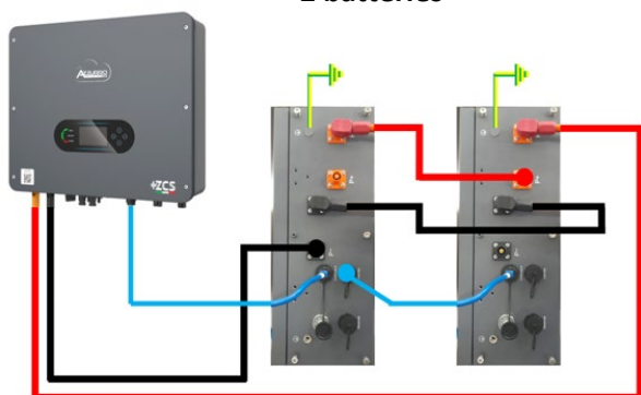
Connexion de 2 batteries
