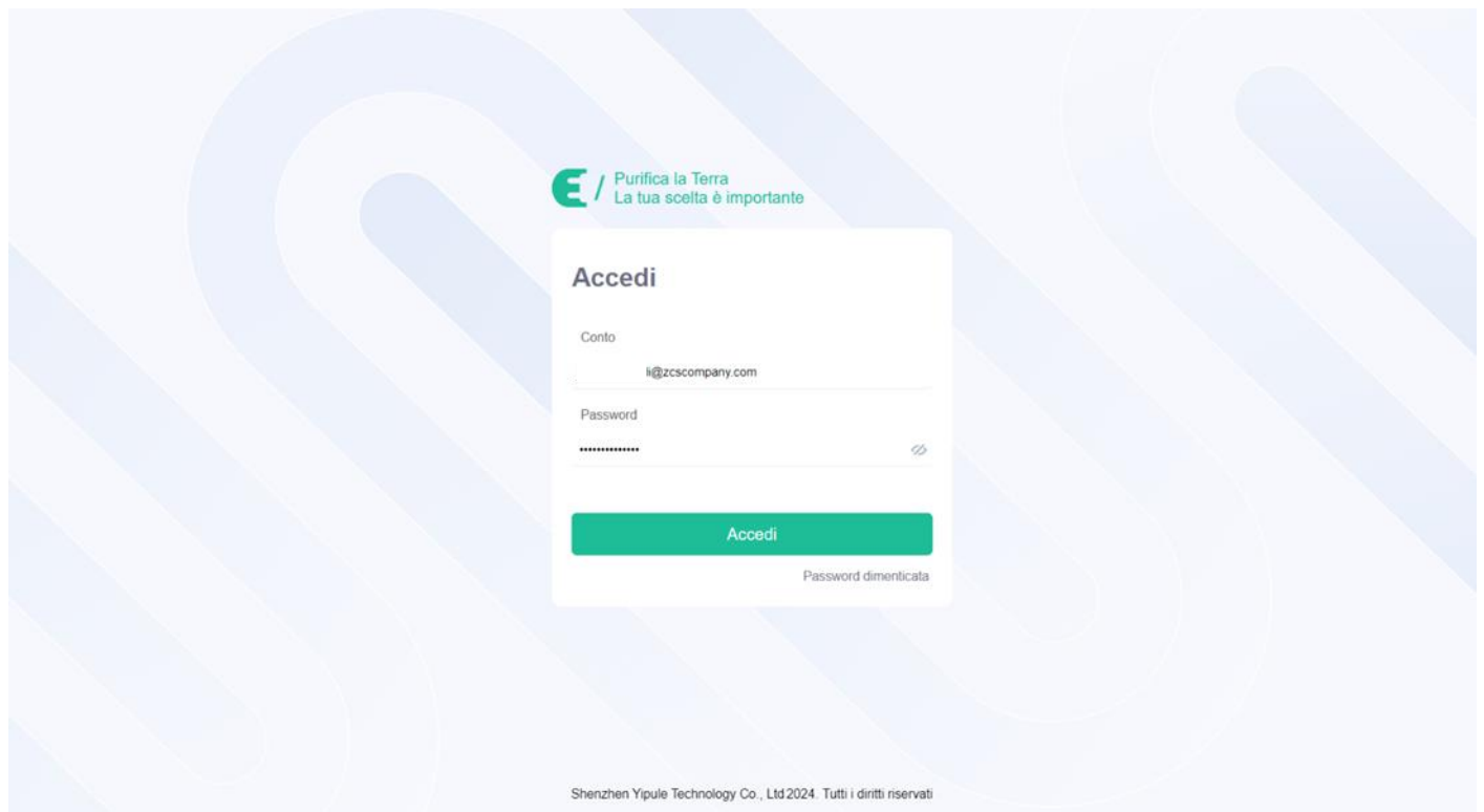
Малюнок 1: Логін.
