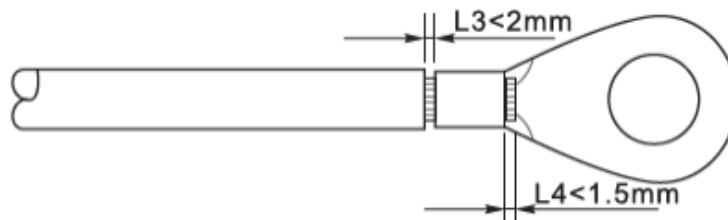
Рис.9 – Підготовка кабелю заземлення (2)
