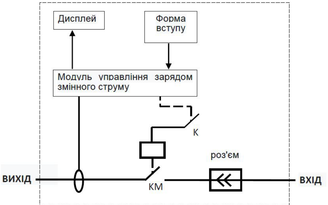
Рис.5 – Схематична робота станції зарядки
