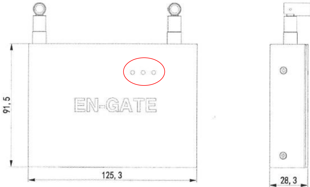
Рисунок 359 - Розміри пристроїв
