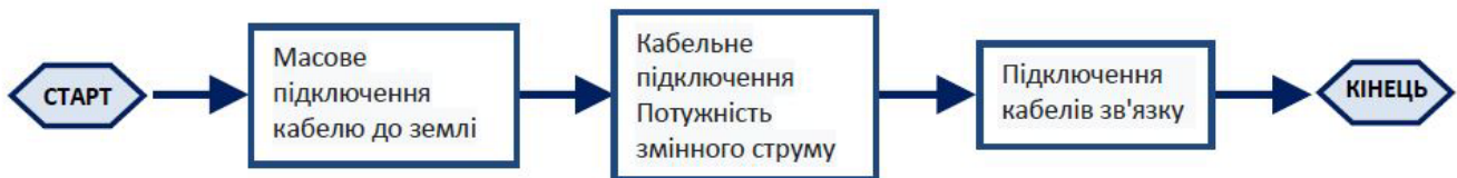
Рис. 7 - Логічна послідовність підключення кабелів
