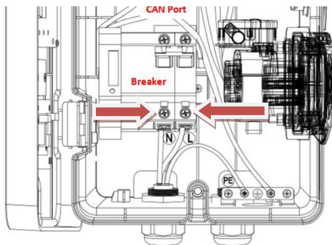
Рис.12 - Підключення вихідних кабелів змінного струму (2)
