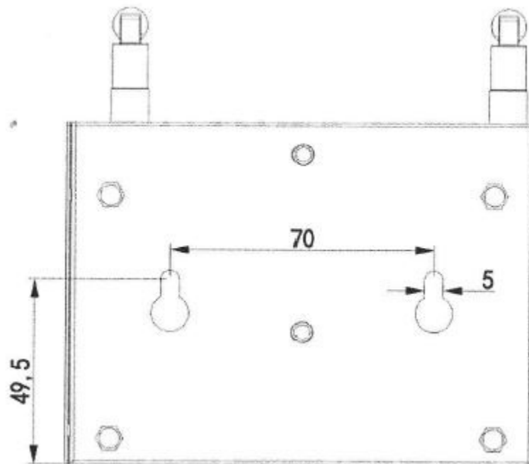
Рисунок 360 - Розміри для встановлення
