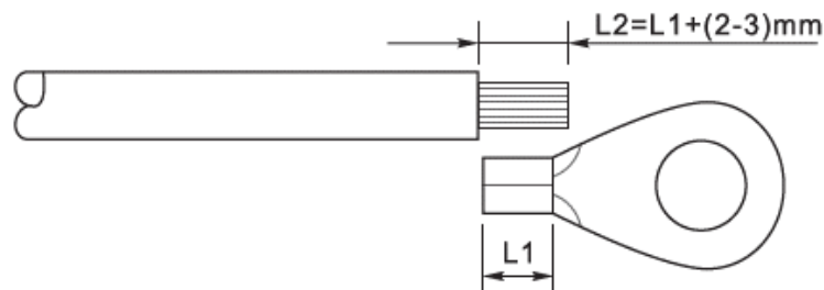
Рис. 8 – Підготовка кабелю заземлення (1)
