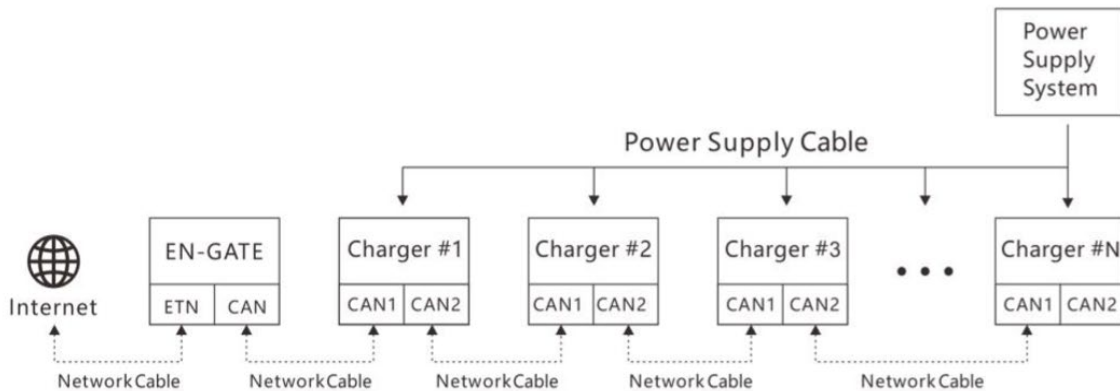
Рис. 15 - Підключення зарядних станцій
