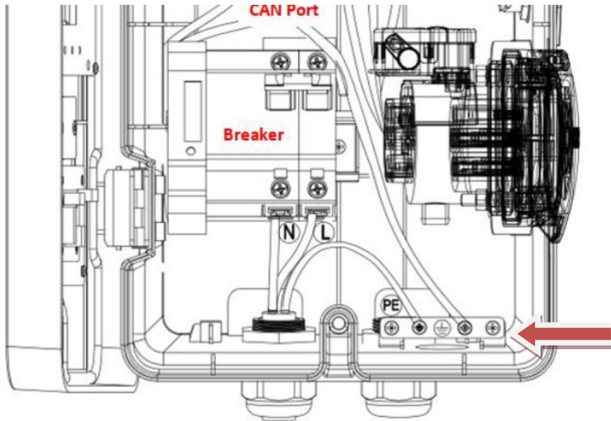
Рис. 10 -- Підключення терміналу заземлення
