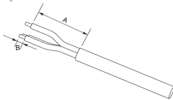
Figura 12 - Podłączenie przewodów wyjściowych zasilania prądem przemiennym (1)
