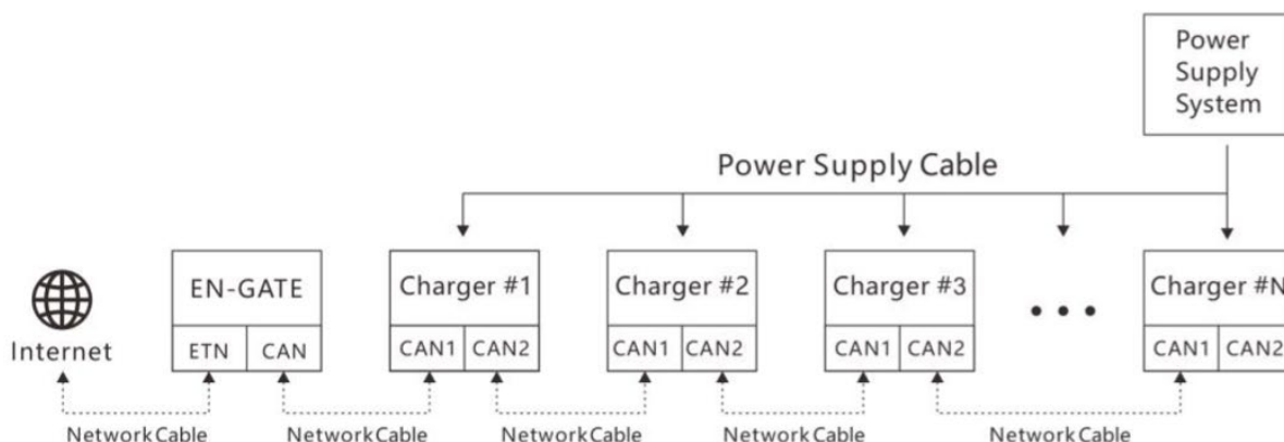
Rysunek 37 - Połączenie między ZVM-GATEWAY a ładowarkami
